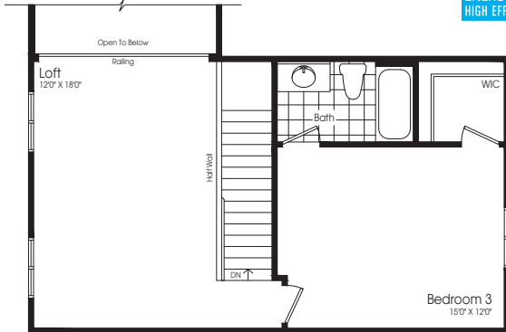
OPTIONAL LOFT FLOOR PLAN 'A'
