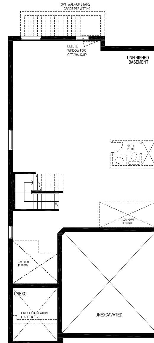
BASEMENT PLAN 'A' & 'B'
