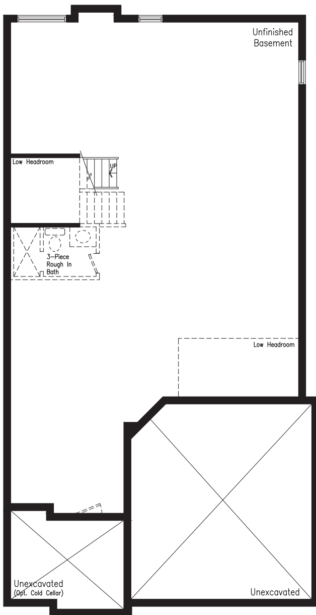
BASEMENT PLAN 'A' & 'B'
